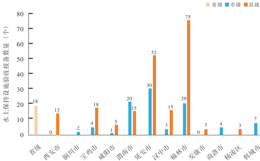
图33 2020年陕西省水土保持设施验收报备数量
