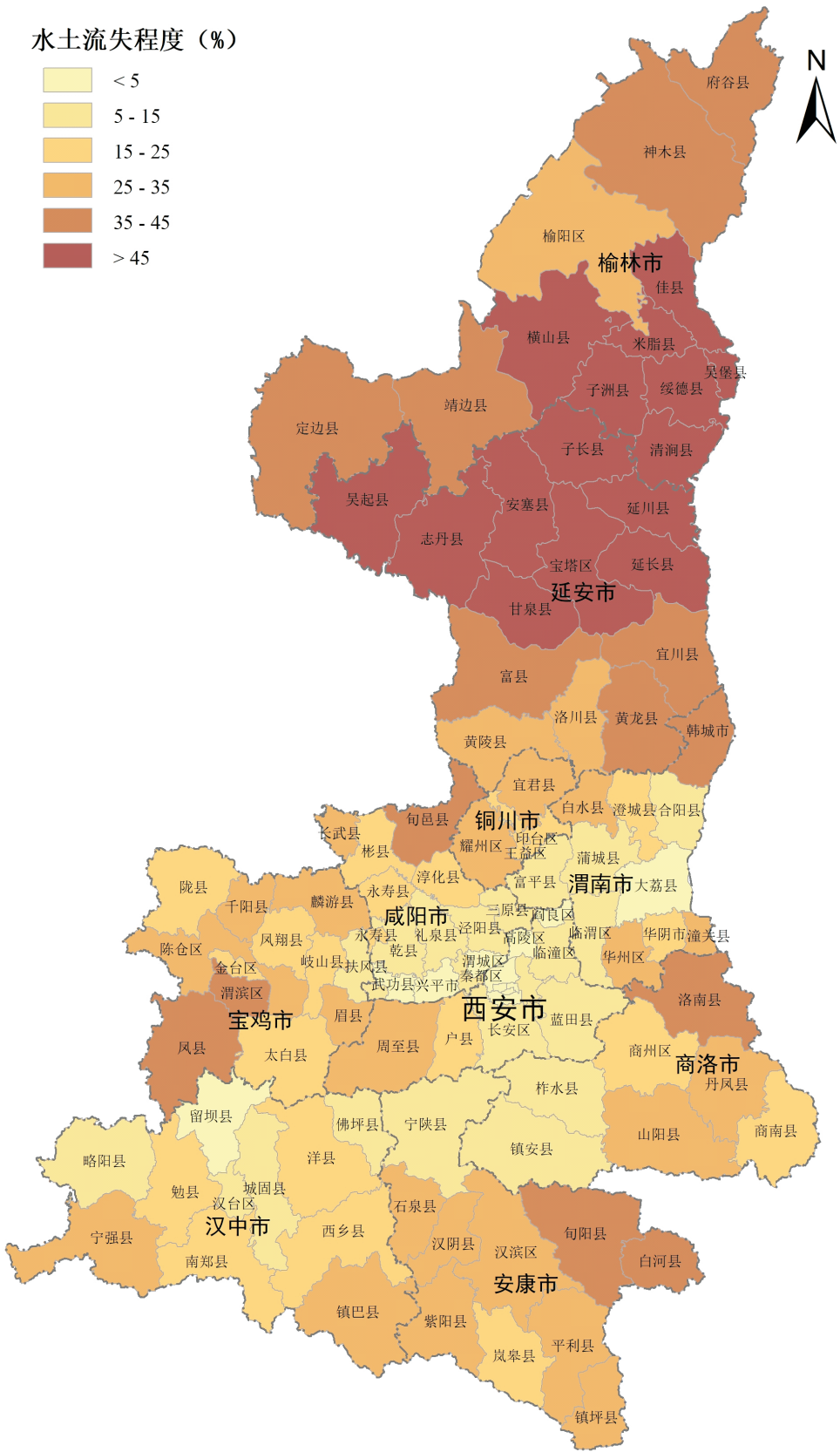
图4 2020年陕西省各县（区）水土流失程度空间分布
