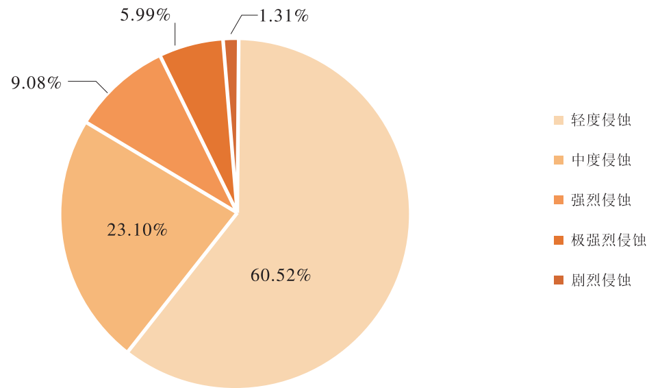
图1 2020年陕西省水土流失面积等级比例
