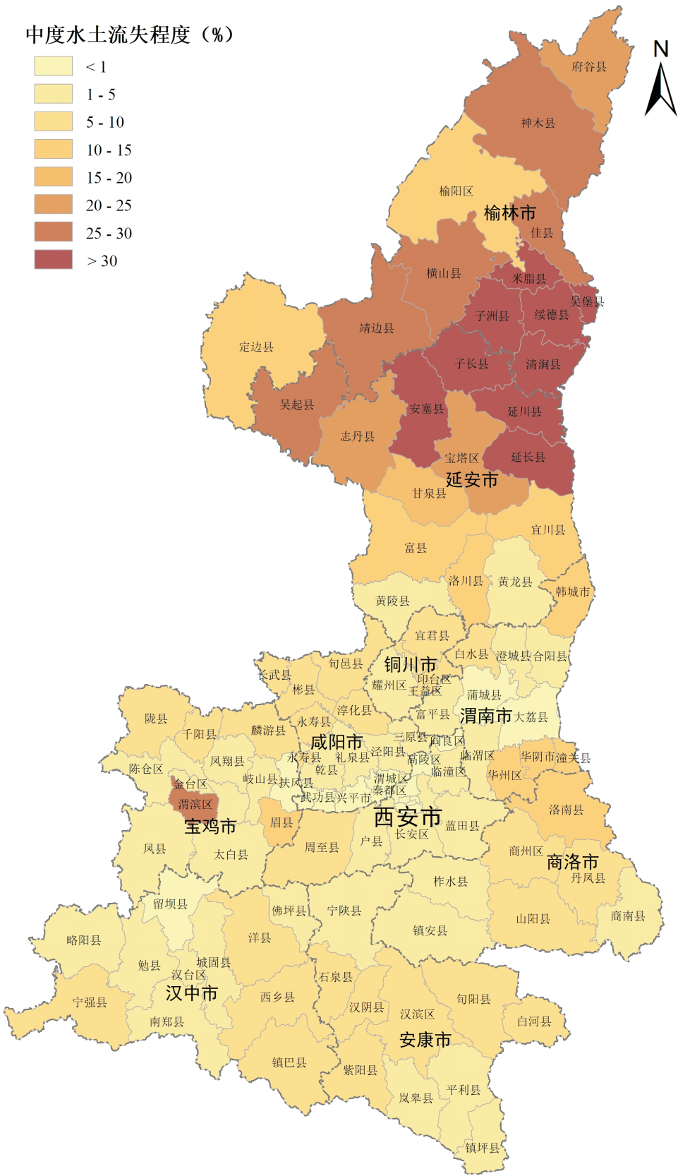
图5 2020年陕西省各县（区）中度水土流失程度空间分布
