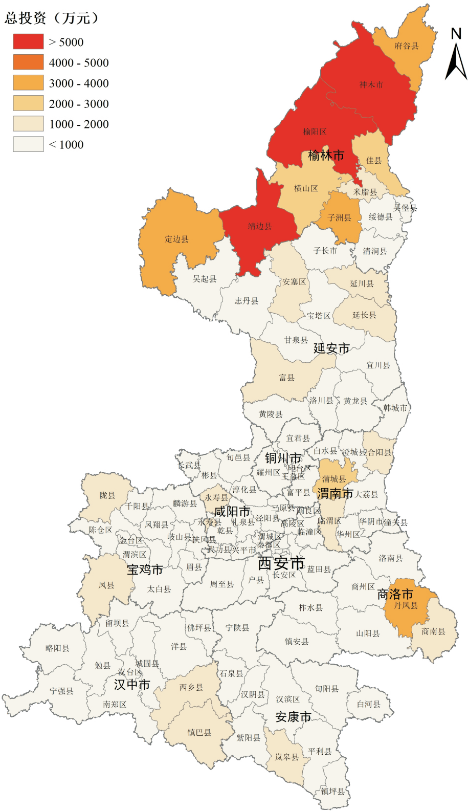
图11 2020年陕西省各县（区）水土保持重点项目投资分布情况
